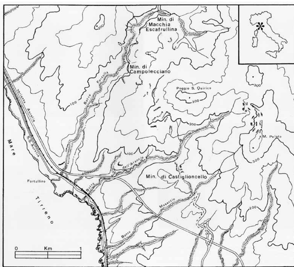
Fig.1: area delle miniere di Masaccio (Castiglioncello), Campolecciano (Fortullino) e Macchia Escafrullina. Da Bracci e Orlandi (1985) 1 .
